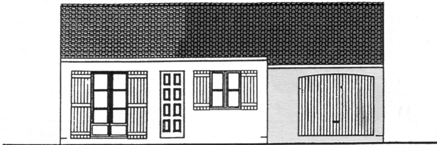
Façade Sud-Ouest
