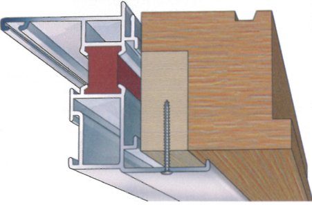
Fixation frontale
