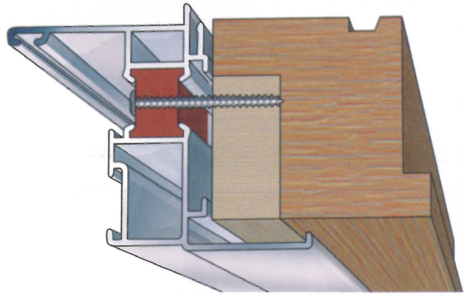
Fixation en feuillure
