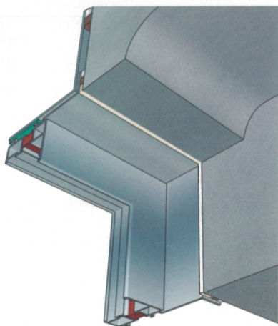
Phase 1 : avant mise en place de la bavette Étanchéité périphérique sur menuiserie aluminium à cadre tournant.
