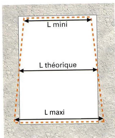
Tolérance 1 cm
