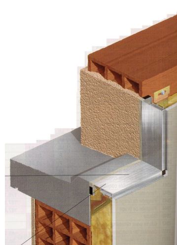
Précadre ALU
